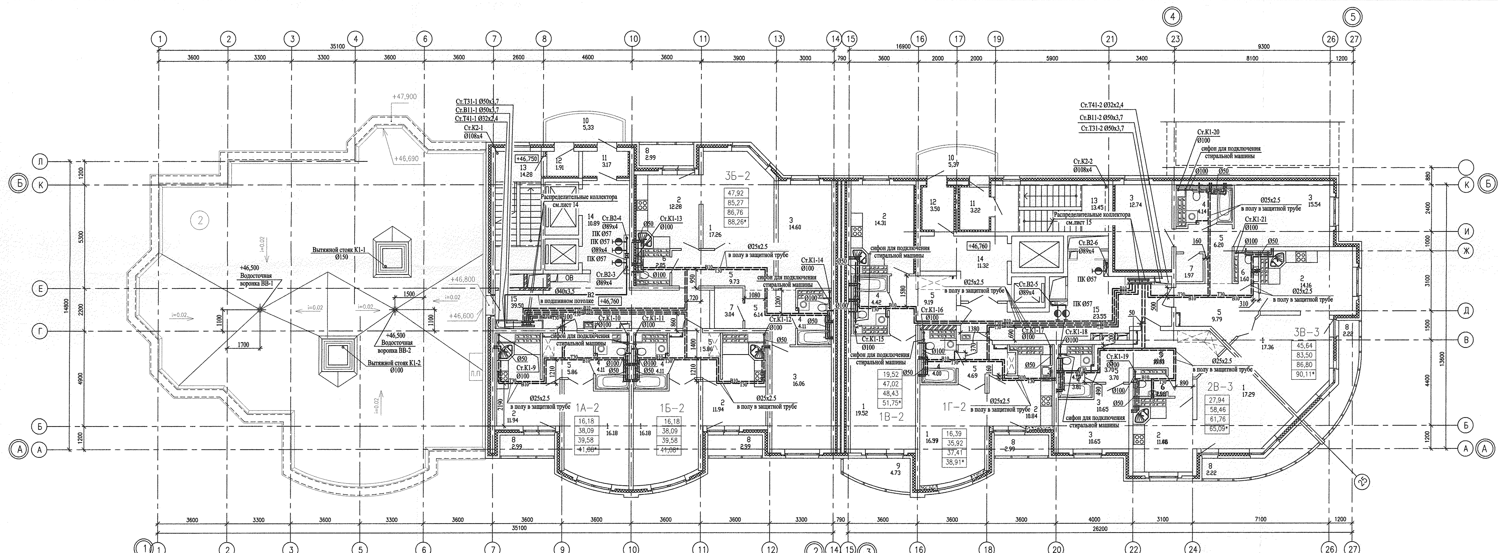
Экспликация помещений
